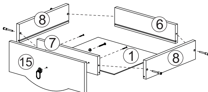
Схема 5а
